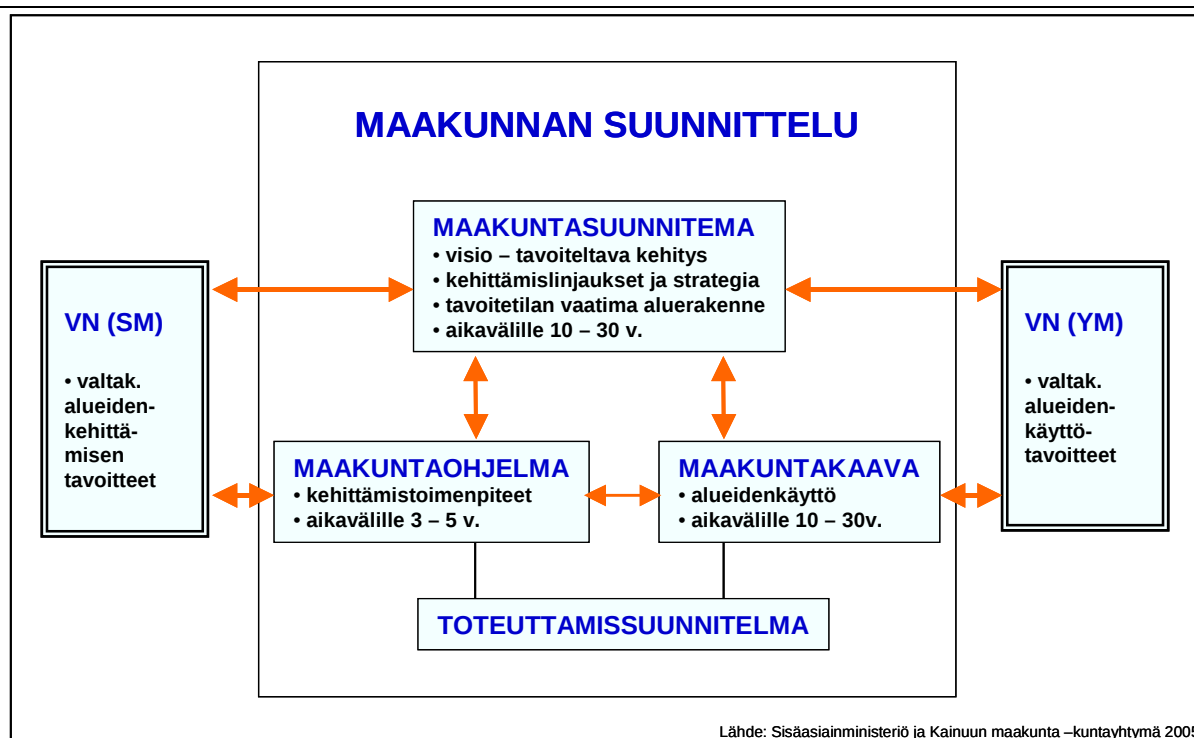
Kuva 3. Maakunnan suunnittelujärjestelmä.
